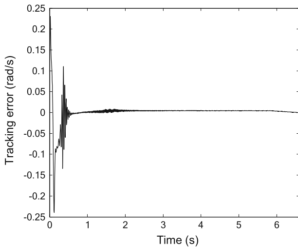
Fig. 10 Trajectory tracking error
