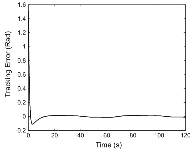
Fig. 4 Trajectory tracking error
